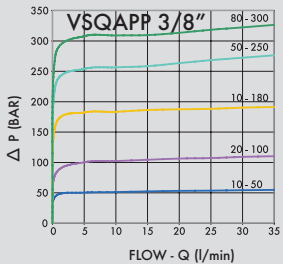
PRESSIONE/PORTATA PRESSURE/FLOW
