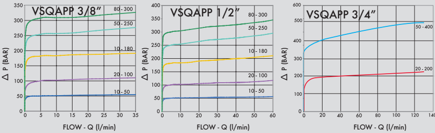
PRESSIONE/PORTATA PRESSURE/FLOW
